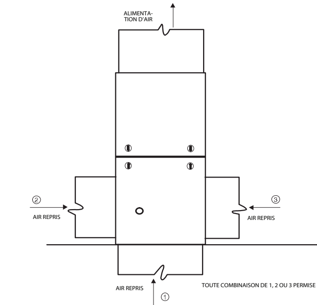
Fig. 21 – Configurations et restrictions de l'air de retour ascendant
