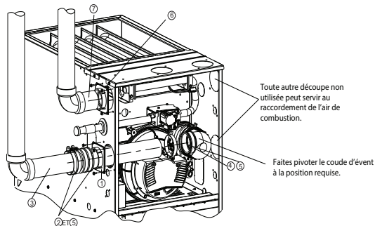
CONFIGURATION À GAUCHE À TIRAGE ASCENDANT
