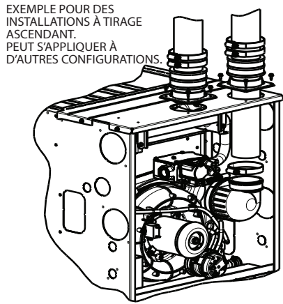
Fig. 44 – Exemple de raccordement de tuyau d'entrée d'air pour des systèmes de ventilation en polypropylène
