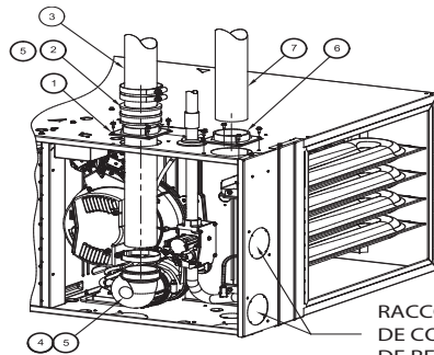
CONFIGURATION HORIZONTALE À DROITE ET VENTILATION VERTICALE
