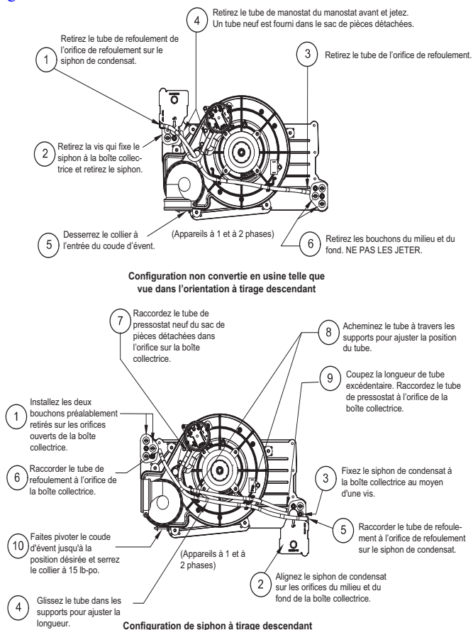
Fig. 9 – Configuration de siphon à tirage descendant (l'apparence peut varier) A11587FR
