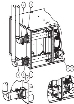
CONFIGURATION HORIZONTALE À DROITE ET VENTILATION VERTICALE
