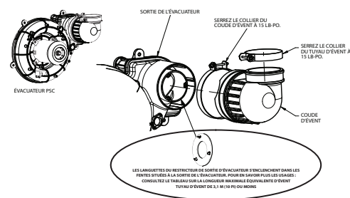
Fig. 53 – Coude d'évent d'évacuateur
