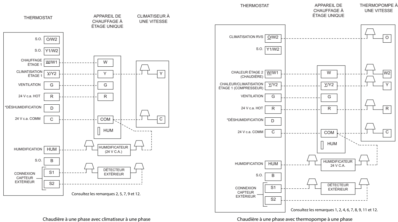
Fig. 39 – Schémas de câblage de thermostat
