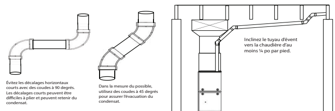
Fig. 52 – Raccordement des événements près de la chaudière
