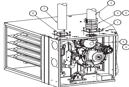
CONFIGURATION HORIZONTALE À GAUCHE ET VENTILATION VERTICALE
