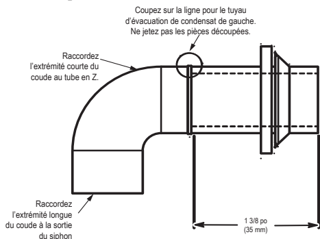
Fig. 17 – Modification du coude d'évacuation en caoutchouc
