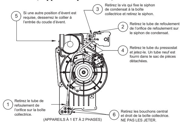
Fig. 10 – Configuration de siphon horizontal à droite (l'apparence peut varier) A11573FR
