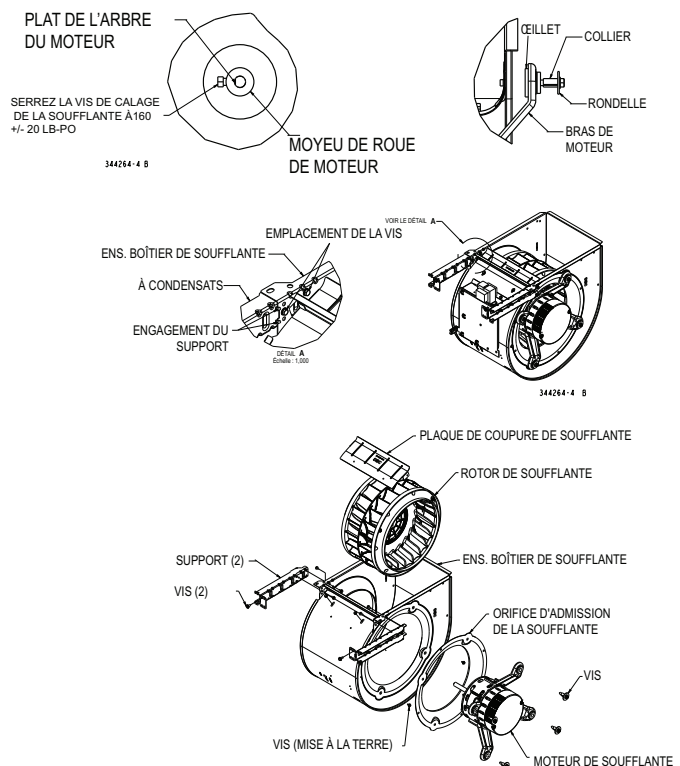
Fig. 65 – Ventilateur en marche 040E14--10 et 060E14--12
