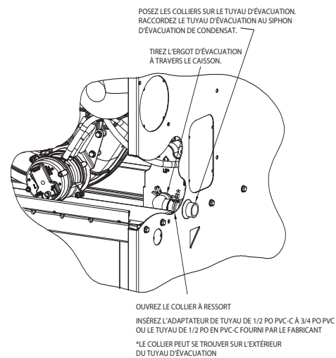
INSTALLATION AVEC ÉVACUATION À DROITE
