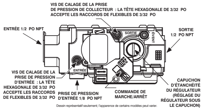
Fig. 63 – Soupapes de gaz
