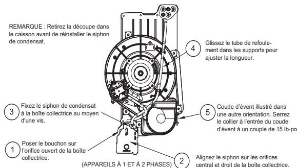
Fig. 10 – Configuration de siphon horizontal à droite (l'apparence peut varier) A11573FR
