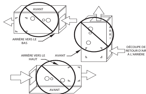
Fig. 4 – Installations prohibées
