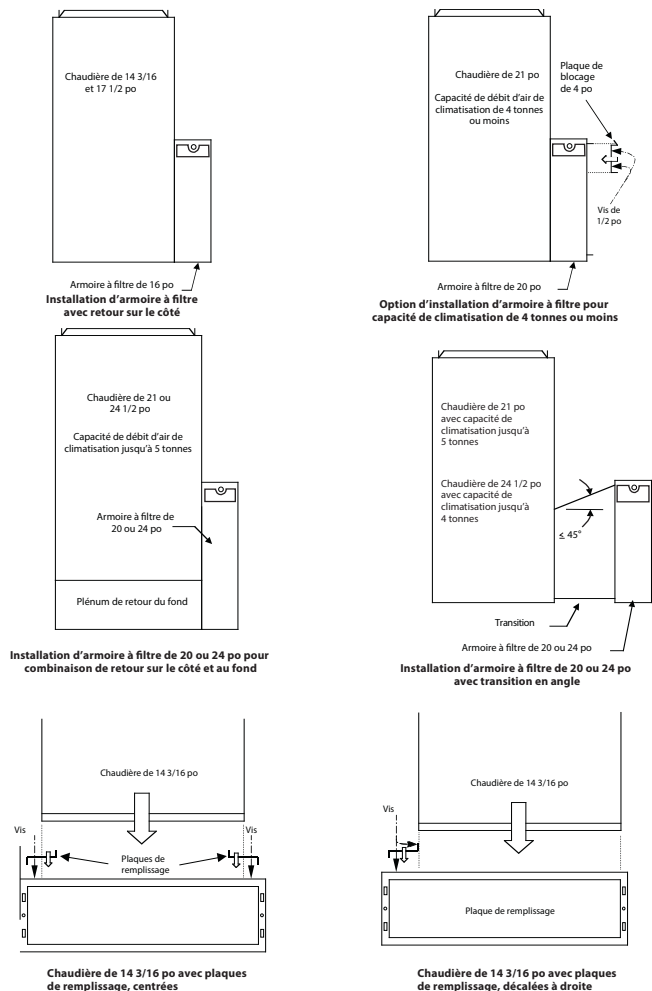
Fig. 26 – Accessoire pour armoire milieu filtrant en option
