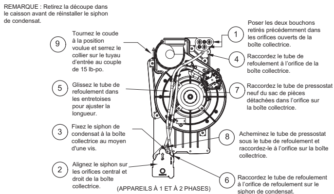
Fig. 11 – Configuration horizontale gauche (l'apparence peut varier) A11574FR
