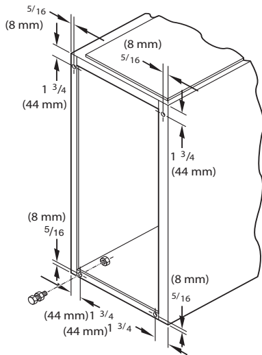
Fig. 29 – Pattes de mise à niveau
